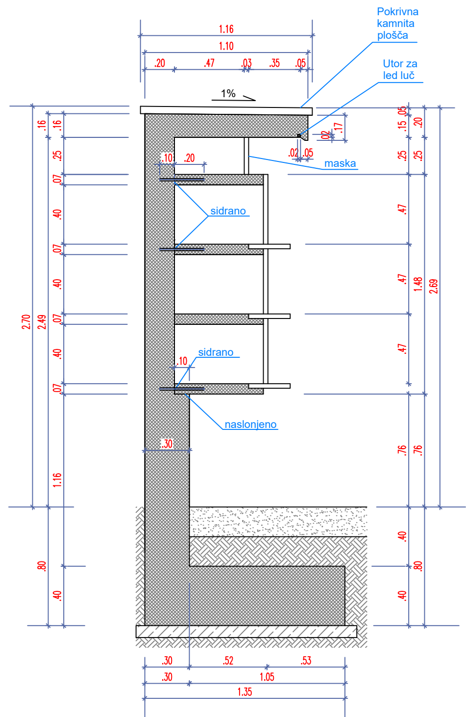
PREREZ ŽARNEGA ZIDU, MERILO M 1:25
