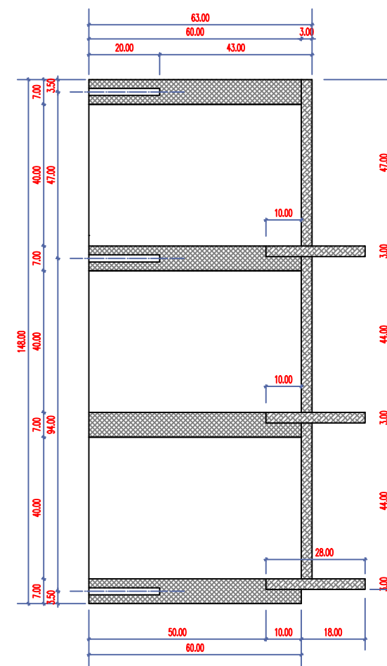
DETAJL ŽARNE NIŠE, MERILO M 1:15
